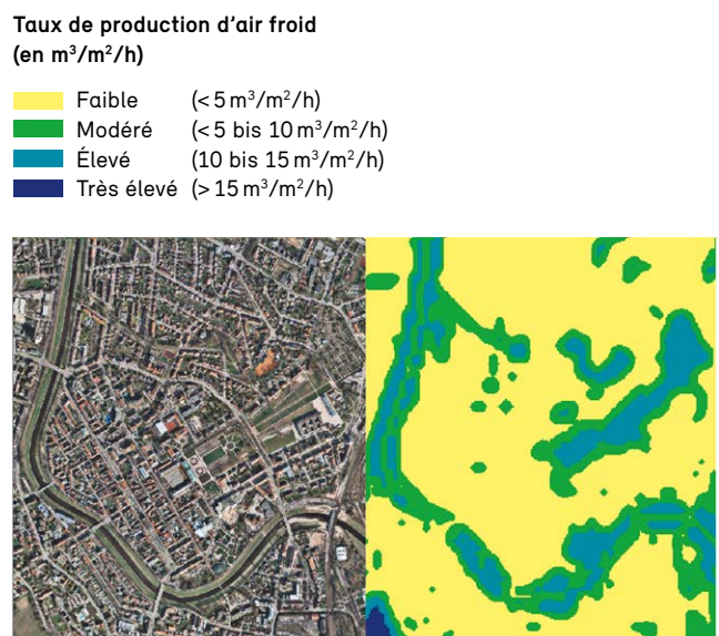
Fig. 29 : Taux de production d'air froid dans le centre-ville de Rastatt en lien avec l'utilisation du sol (détail)
