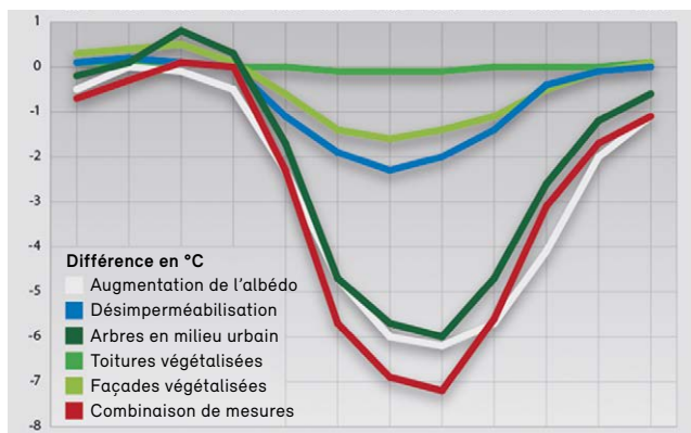
Figure 92 Évaluation des conséquences de différentes variantes de plans (A et B) sur le climat pour un projet résidentiel à Ettlingen
