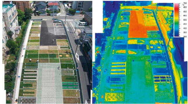
Fig. 81 : Température en fonction du matériau de surface. Parking expérimental à Kobe. Mesure à 21h
