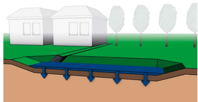
Figure 61 Schéma d'une dépression d'infiltration avec écoulement et espace de rétention en surface
