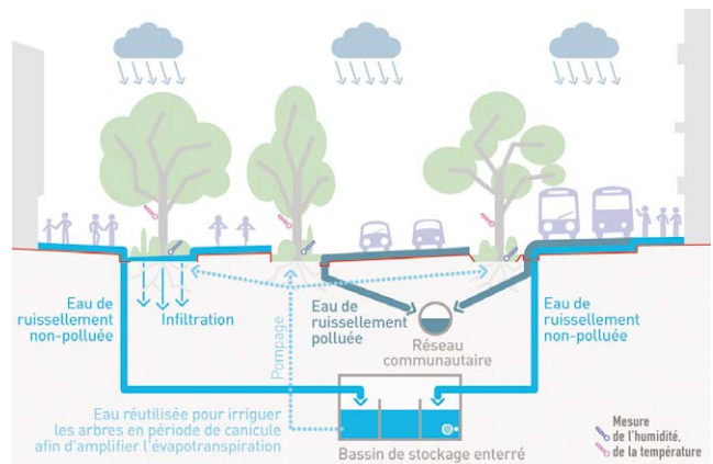
Figure 67 Système de stockage et d'irrigation, rue Garibaldi à Lyon
