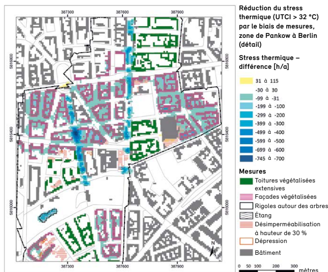
Figure 16 Modélisation à micro-échelle avec ASMUS (résolution de 8 m) dans le cadre du projet de recherche KURAS pour le site modèle de Pankow, Berlin
