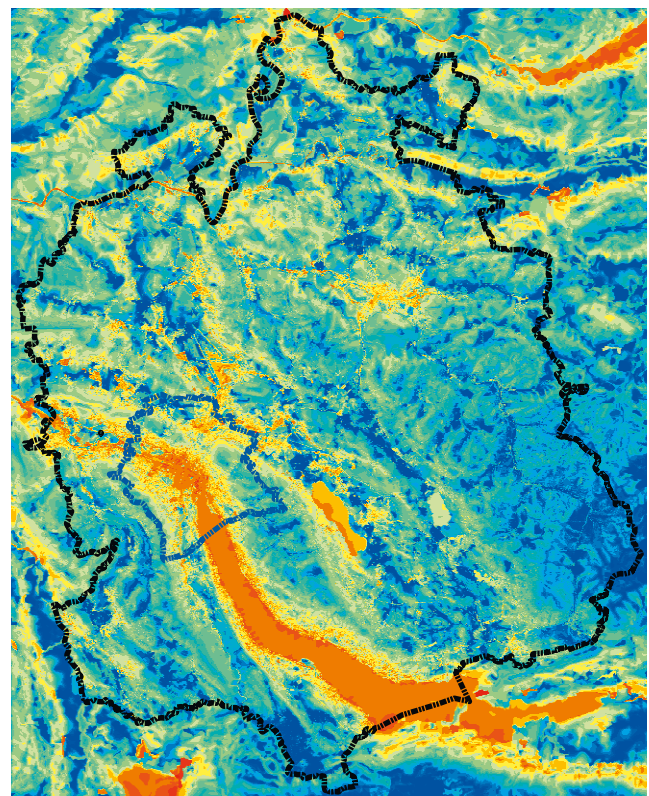
Figure 5 Température de l'air pendant une nuit d'été à vent faible (à 2 m du sol). Canton de Zurich modélisation avec FITNAH – carte de base de l'analyse climatique.
