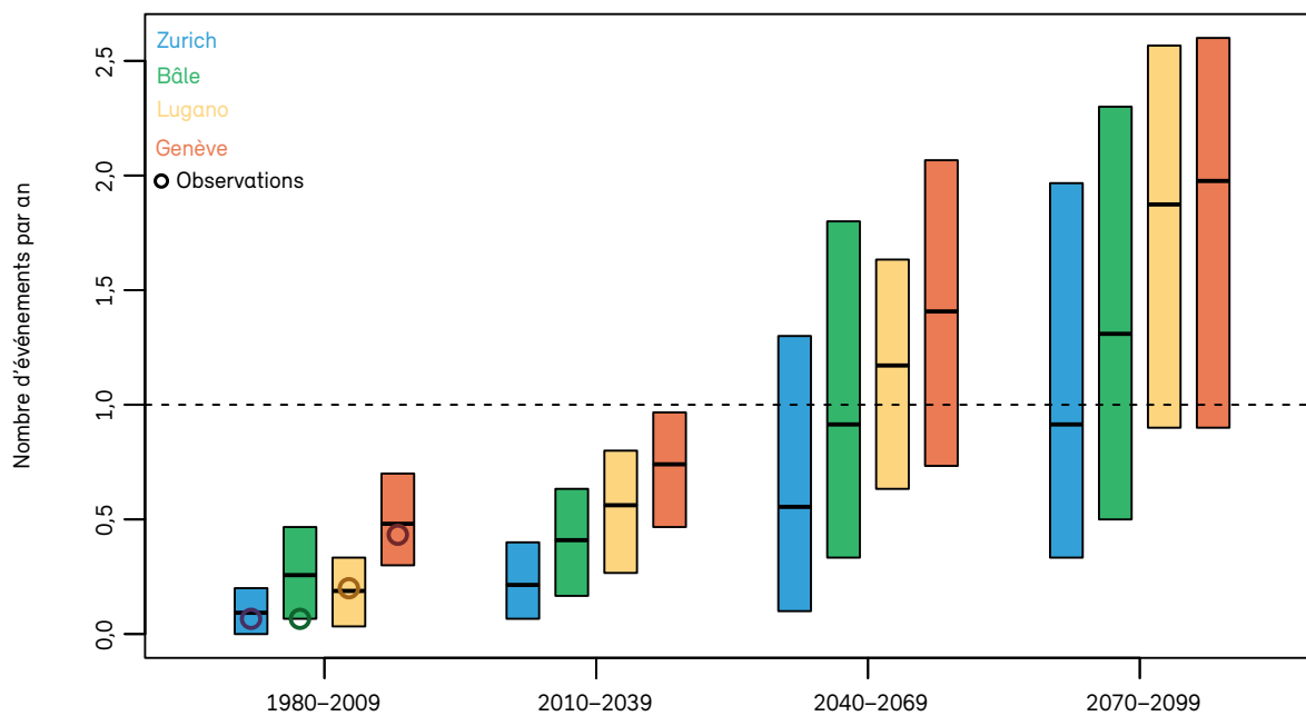
Figure 3 Nombre annuel de vagues de chaleur d'au moins sept jours consécutifs
