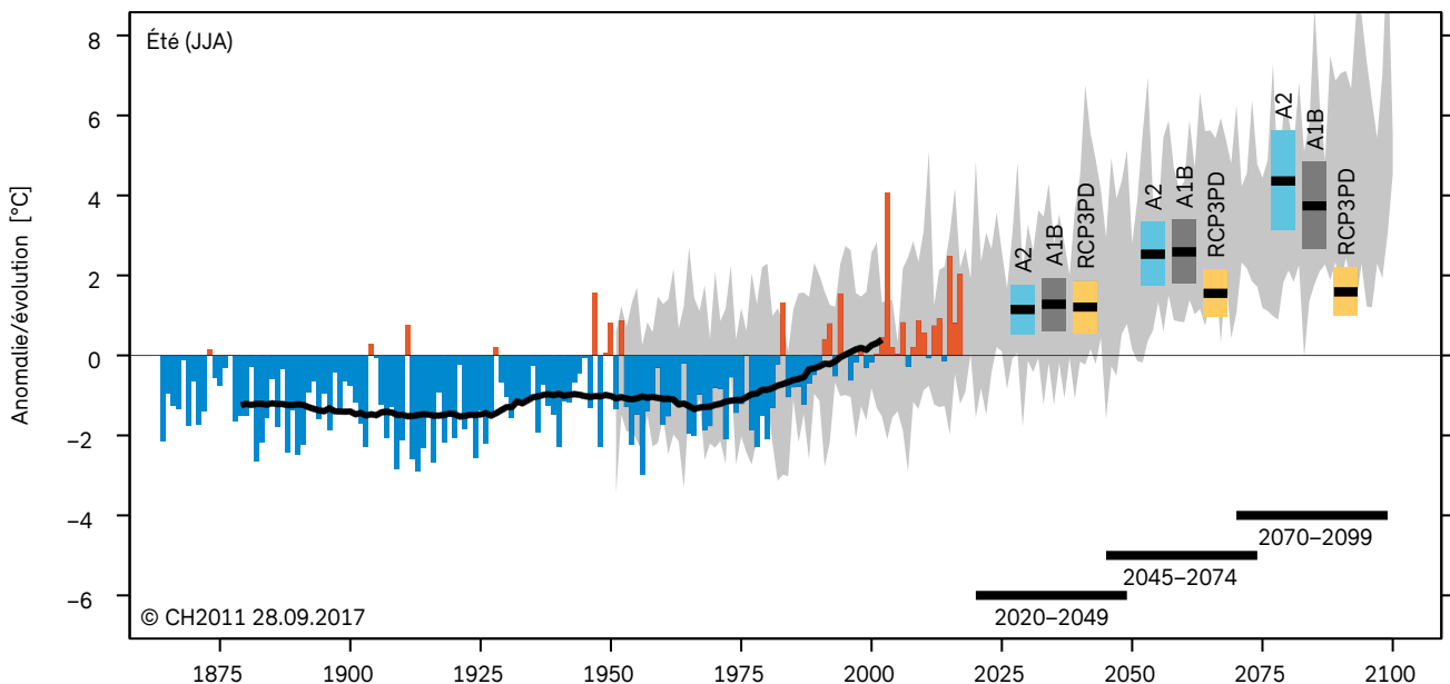
Figure 11 Changements de température passés et futurs pendant les mois d'été A2.6
