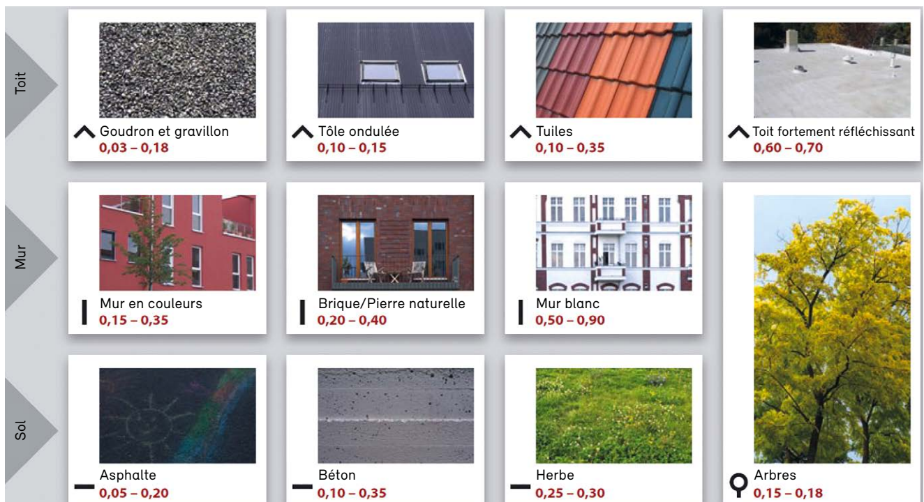
Fig. 80: Valeurs d'albédo de différentes surfaces A3.2
