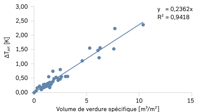
Figure 32 Capacité d'abaissement de la température en fonction du volume de verdure spécifique. Simulation à une hauteur de 1,5 m, vers 14 h
