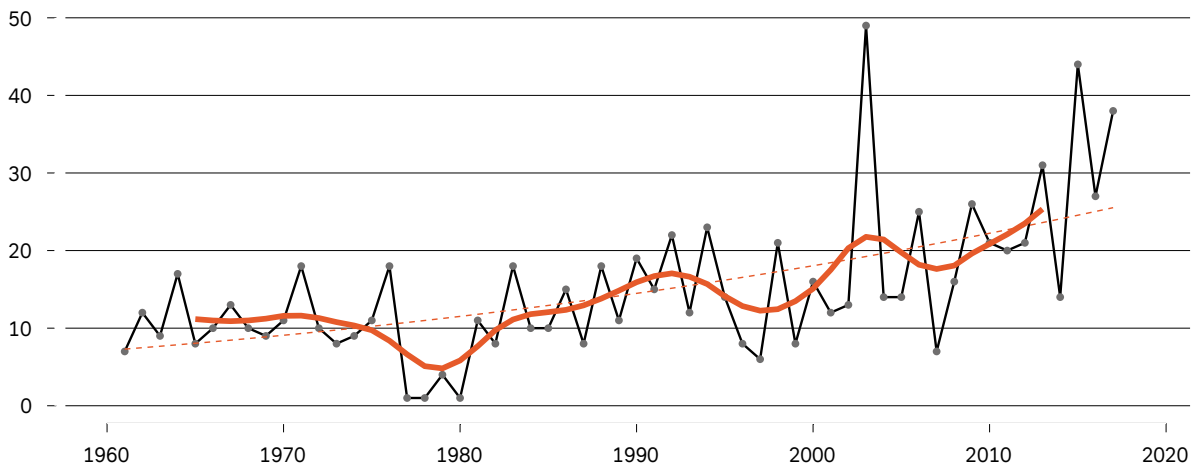
Figure 2 Nombre de jours tropicaux (température \geq 30 °C) à Sion
