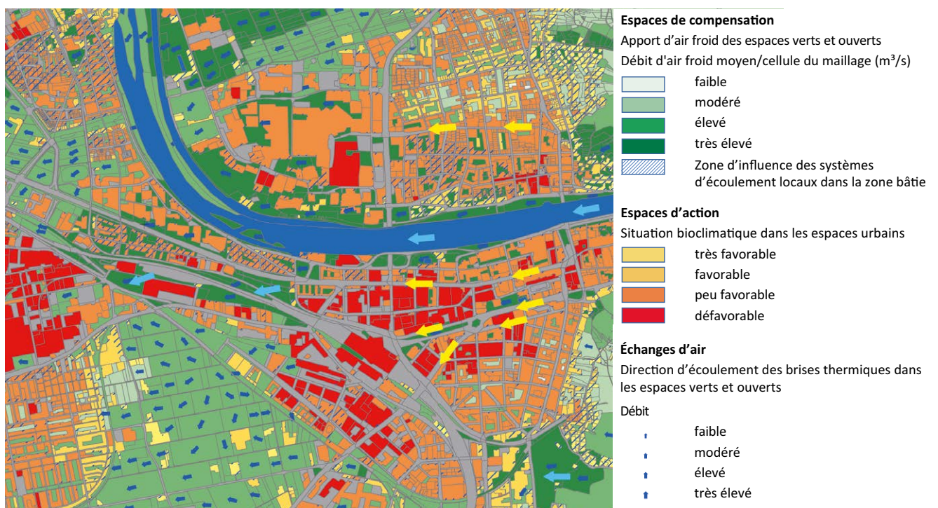
Carte de l'analyse climatique de la ville de Heidelberg (détail), sur la base des résultats d'une modélisation à méso-échelle avec FITNAH A3,16
