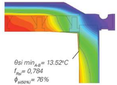
Fig. 54 Illustration des températures au raccord de la dalle des combles et de la façade dans l'étude de cas 03.
