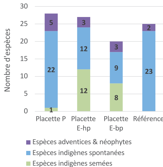
Fig. 3. (a) Taux de recouvrement relevés en 2017 (b) Richesse spécifique relevée de 2015 à 2017 sur l'ensemble des placettes et au sein du milieu naturel de référence
