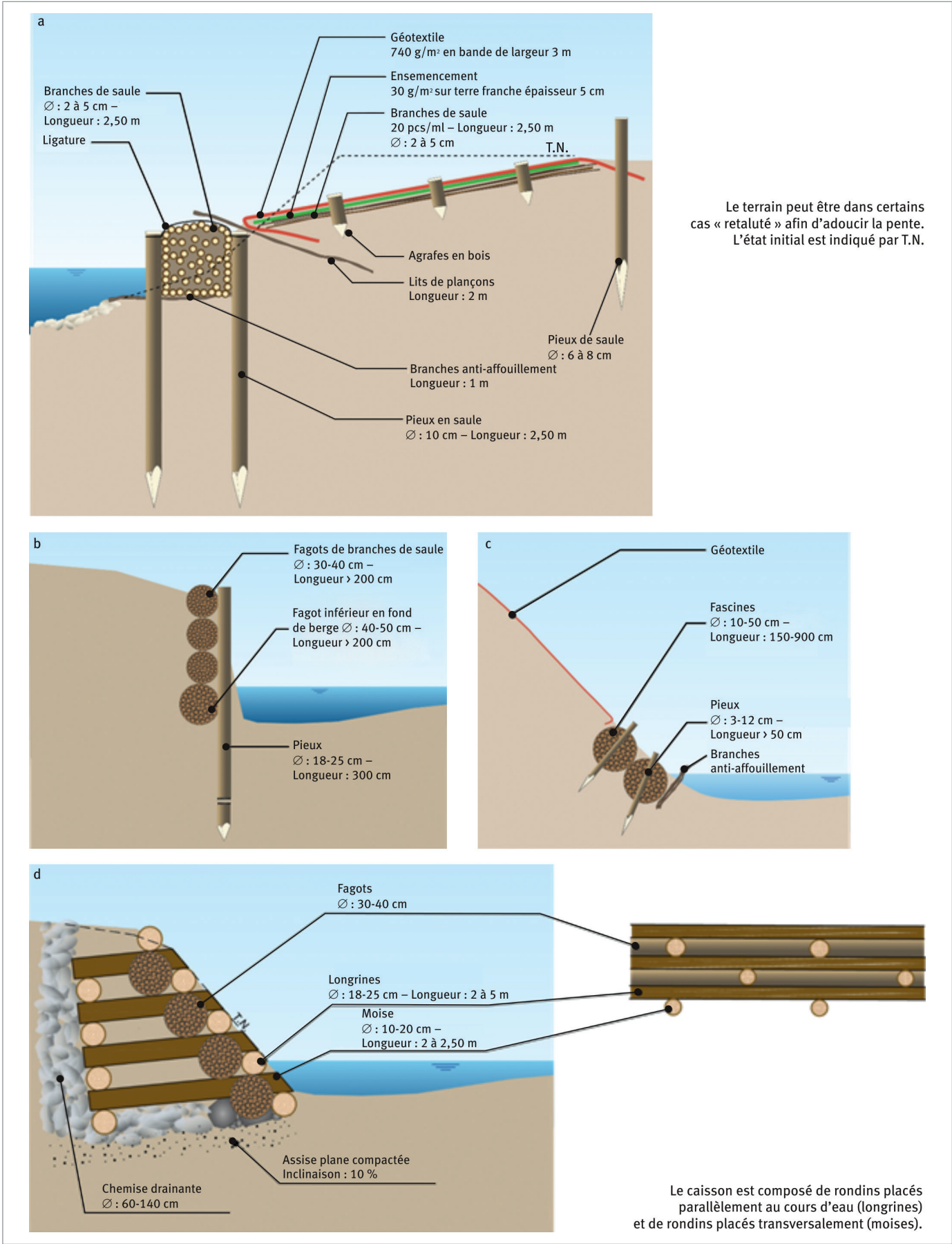
Figure 1 – Profils d'ouvrages en fascines : (a) Fascine en pied de berge, (b) Mur en fascines, (c) Fascines de pente multiples et (d) Caisson avec fascines.
