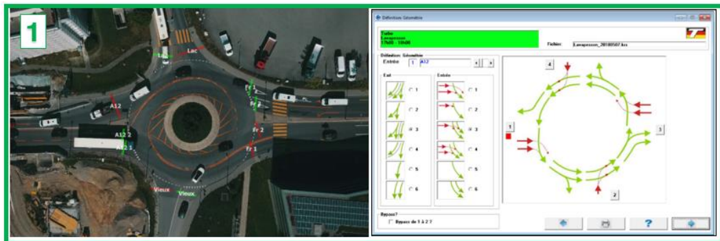
Fig. 103 Lavapesson – Modélisation de l'affectation des voies – Turbo-Kreisverkehr 2015.
