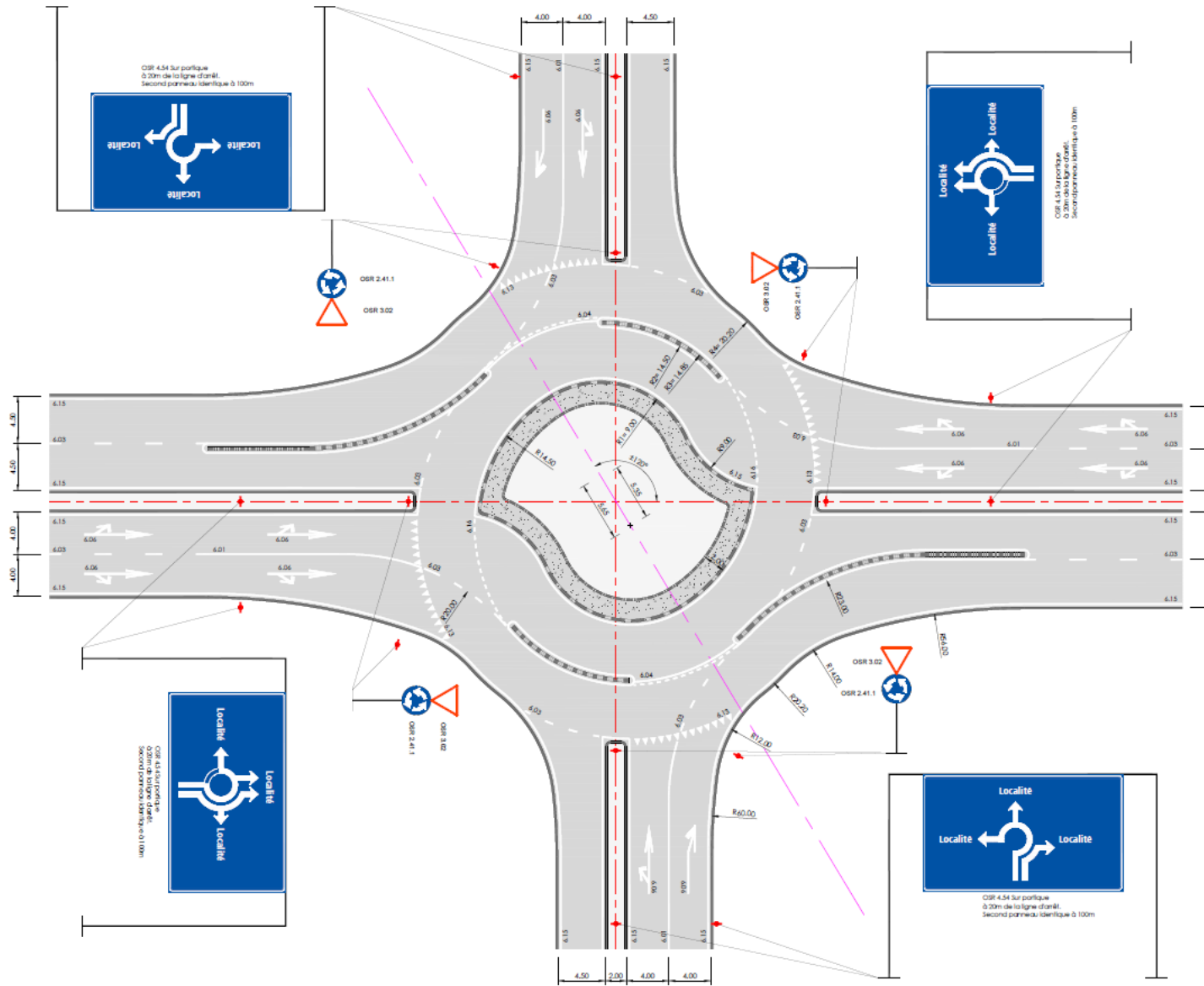
Fig. 45 Turbo-giratoire à quatre branches, diamètre 40m, selon méthode de dimensionnement géométrique adaptée à la Suisse.
