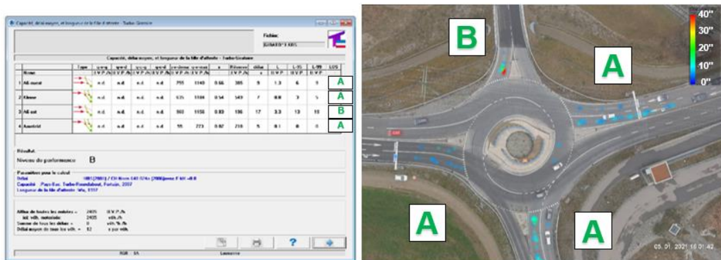
Fig. 98 Glättimüli – Niveau de service – Turbo-Roundabout, Fortuijn, 2007.
