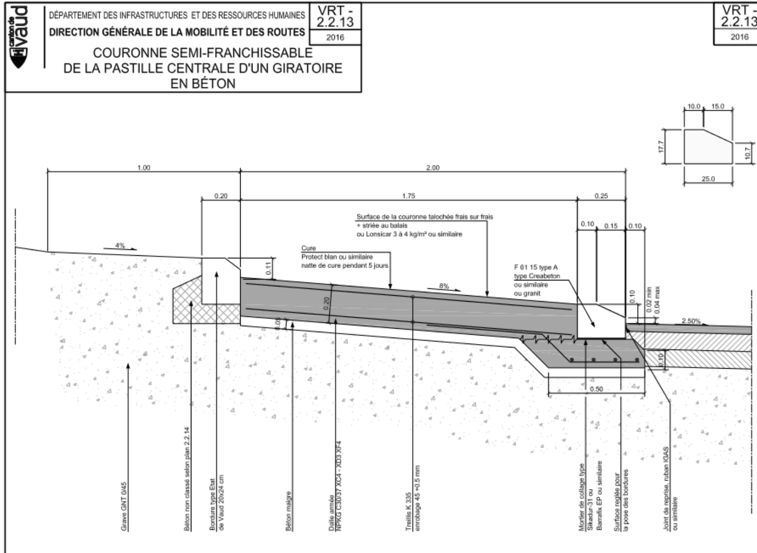
Fig. 41 Détail technique – Surface semi-franchissable en béton, DGMR, Canton de Vaud.
