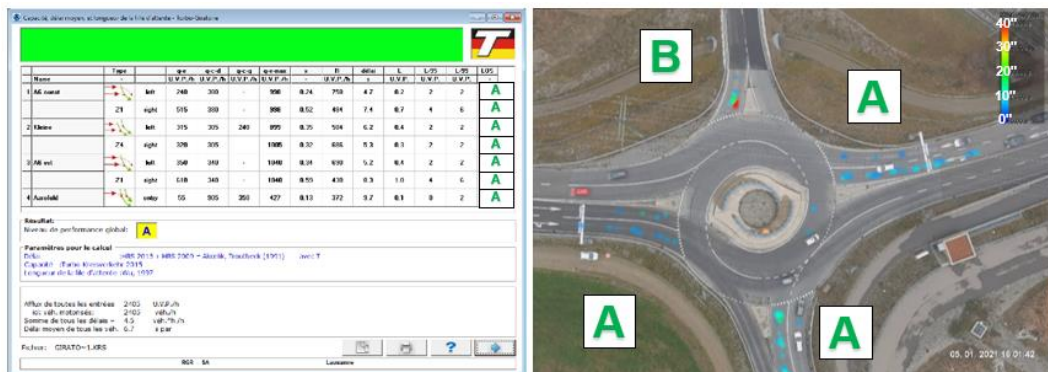
Fig. 92 Glättimüli – Niveau de service – Turbo-Kreisverkehr 2015.
