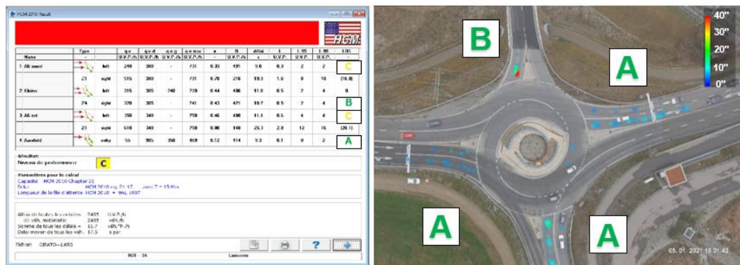
Fig. 101 Glättimüli – Niveau de service – Turbo-Roundabout, Fortuijn, 2007
