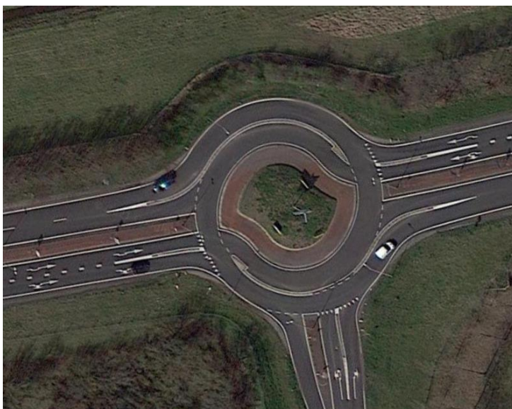
Fig. 82 Turbo-giratoire à 3 branches, Zoetermeer, Pays-Bas, Google Maps, 2021.
